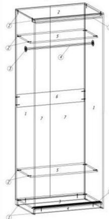
Схема сборки.
