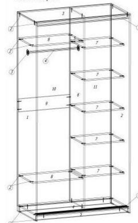
Схема сборки.
