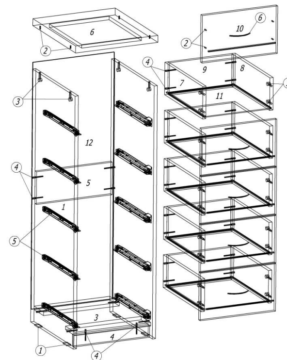
Схема сборки
