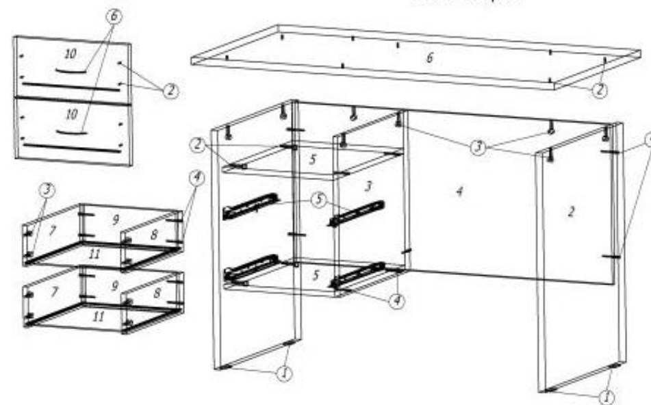
Схема сборки
