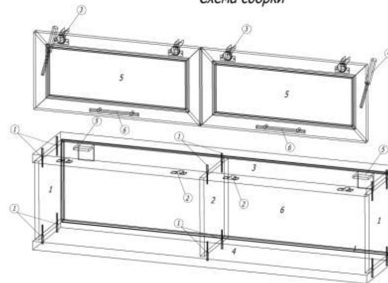
Схема сборки
