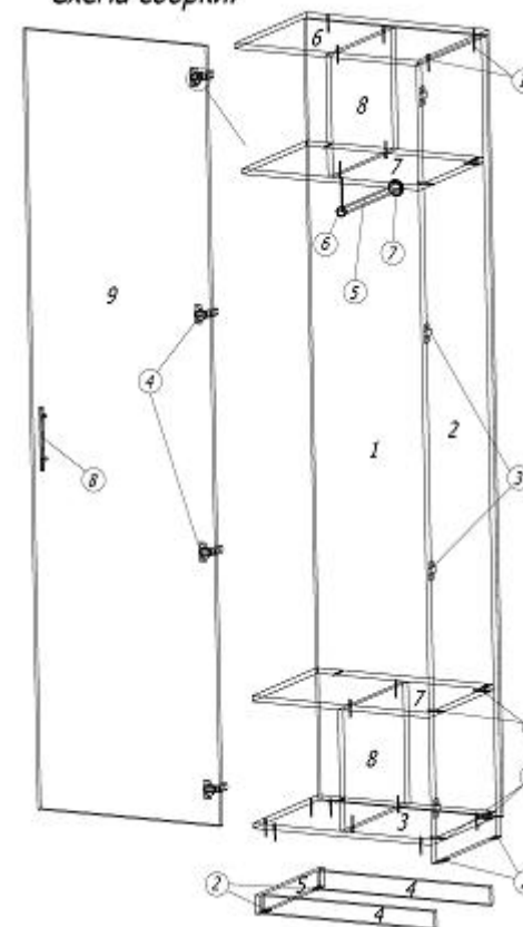
Схема сборки.
