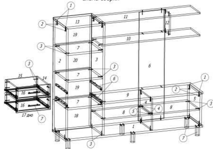
Схема сборки
